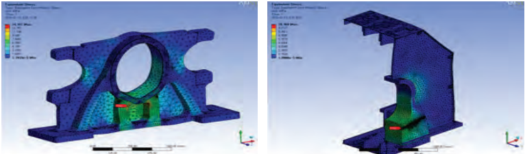
고하중을 고려한 구조해석 시뮬레이션
